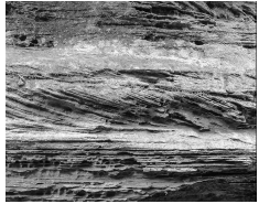
(나) 사층리
